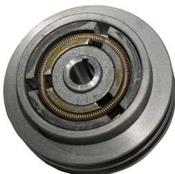
EMBRAGUE PLANCHA C-160
