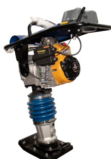
VIBROAPISIONADOR ROBIN SUBARU 4HP POTENCIA: 4HP PESO: 75KG ENCENDIDO MANUAL REVOLUCIONES: 640-700 RPM PROCEDENCIA: JAPAN
