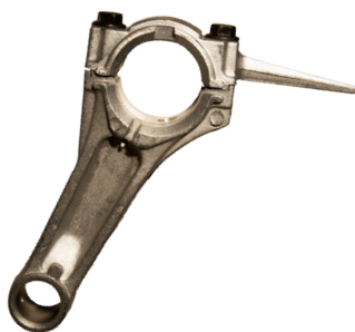
BRAZO DE BIELA HONDA GX160
