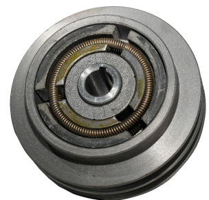
EMBRAGUE PLANCHA C-100
