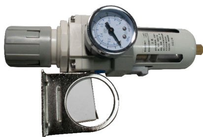
EQUIPO DE MANTENIMIENTO DE 1 VASO 3/8"
