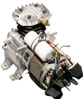
CABEZAL Y MOTOR DIRECTO 2HP
