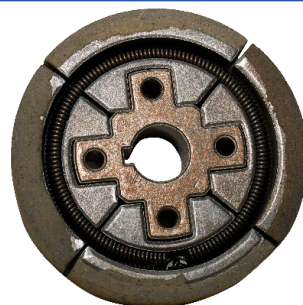
EMBRAGUE DEL VIBROAPISIONADOR ROBIN SUBARU
